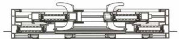
OXXO (4-Panel)
