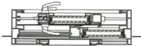
Door Section XO/OX
